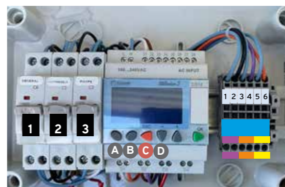
Connexions au tableau électrique.
